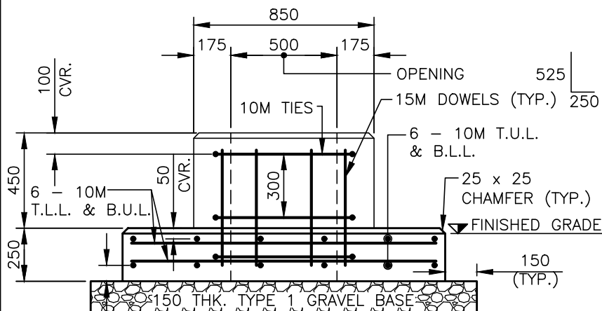
E2 ELEVATION 1:25
