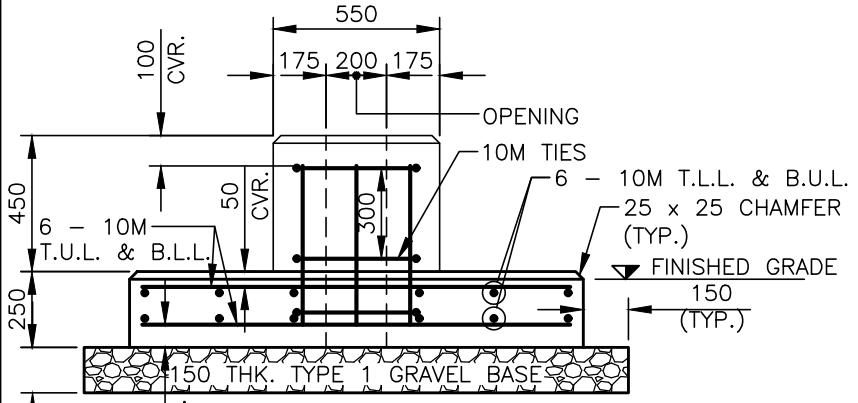
E1 ELEVATION 1:25
